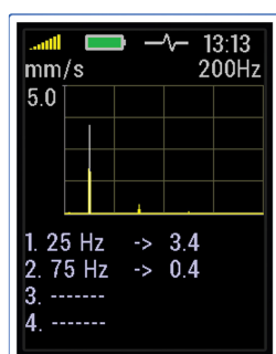
Widmo FFT
